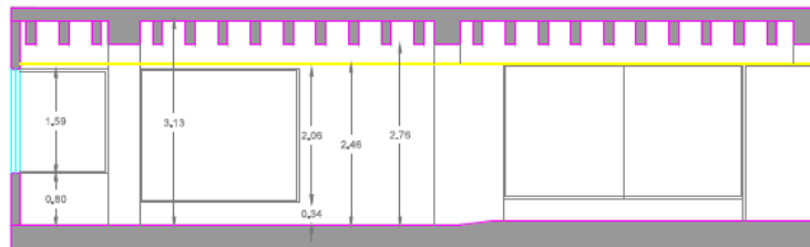
CORTE LONGITUDINAL - B
