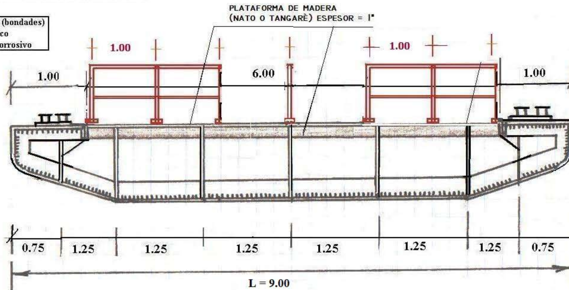
SECCIÓN DEL MODULO AUTO FLOTANTE
