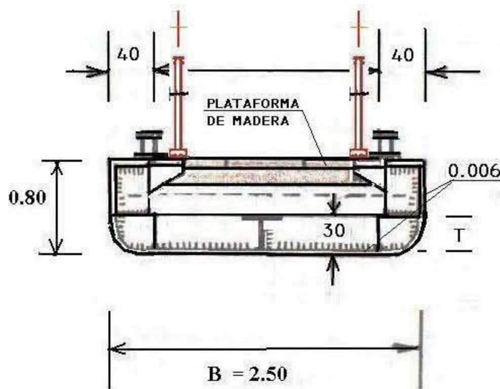
SECCIÓN DEL MODULO AUTO FLOTANTE
