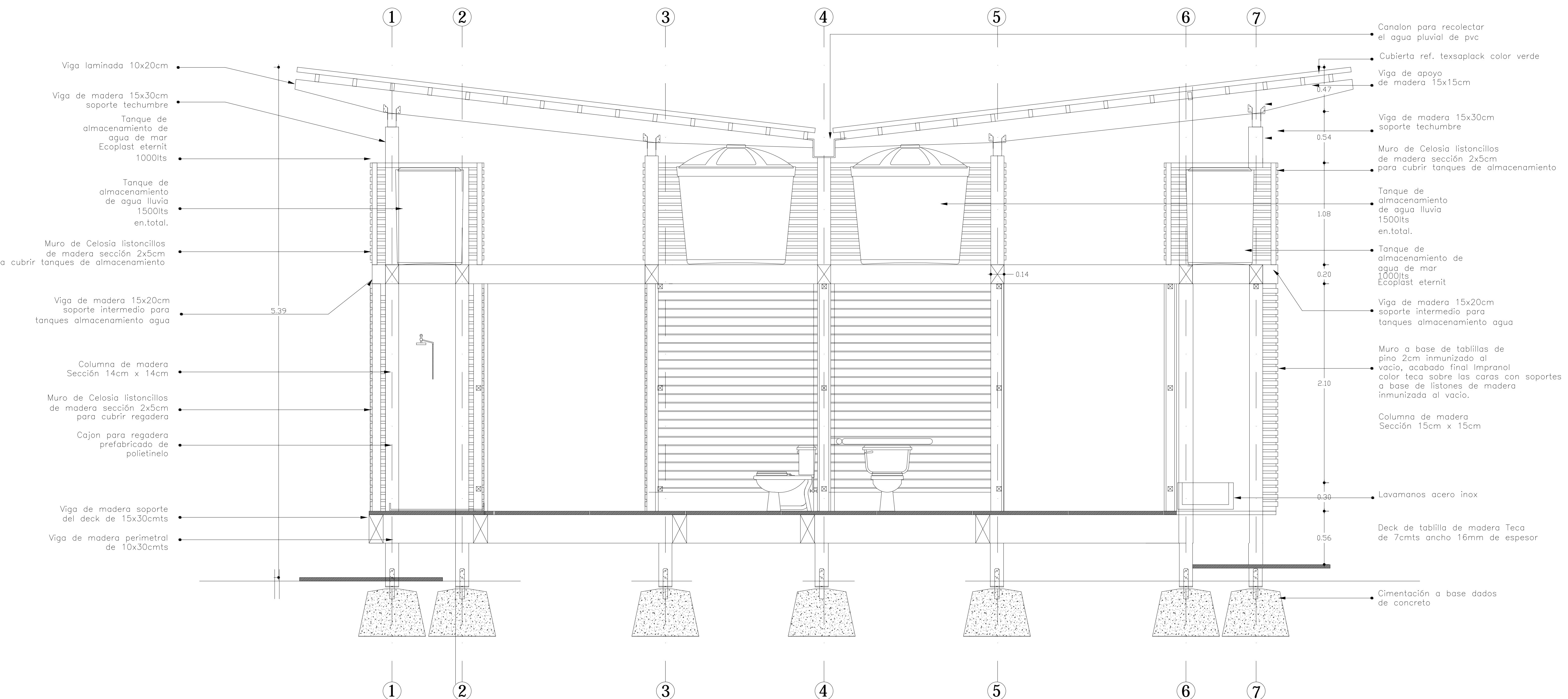
Corte A-A
