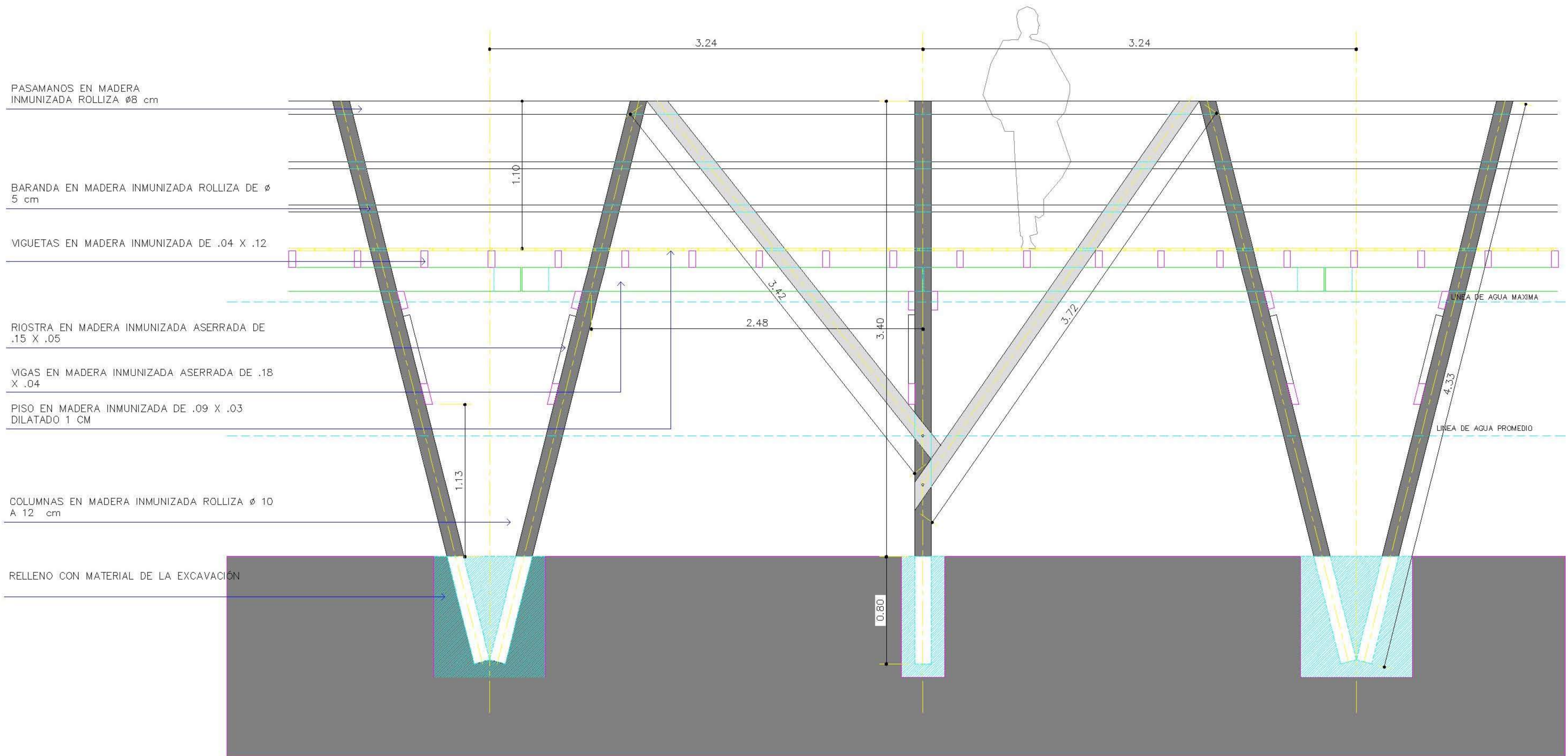
SECCIÓN LONGITUDINAL TRAMO TIPICO
