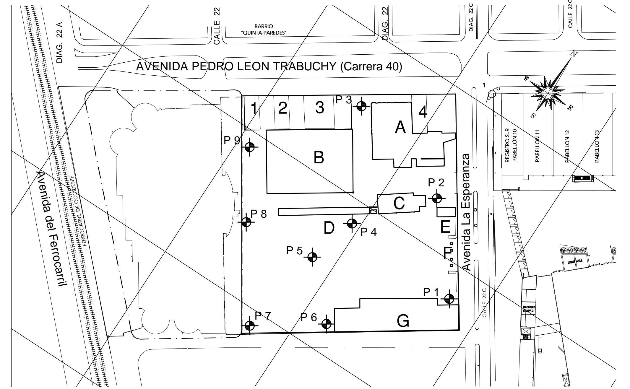
LOCALIZACIÓN DE PERFORACIONES ESC 1: 1500
